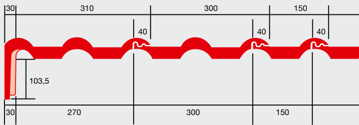
Dekkende breedte linker gevelpan 310 mm.
